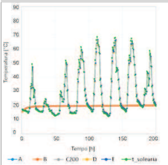
Figura 3 - Milano - Copertura CLS - PU 200 mm
