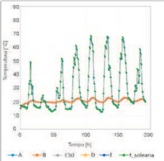
Figura 2 - Milano - Copertura CLS - PU 100 mm
