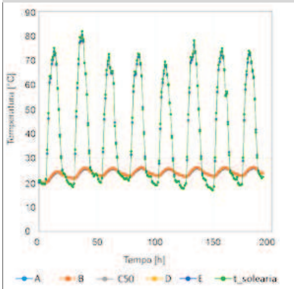
Figura 5 - Palermo - Copertura Laterizio - PU 100 mm
