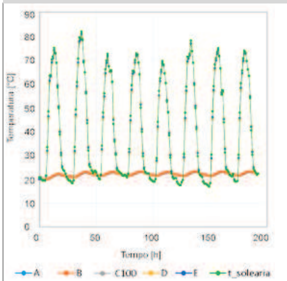
Figura 6 - Palermo - Copertura Laterizio - PU 200 mm
